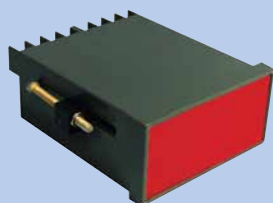
Modelo: AP 48 x 96/8T - Código: 488T/00/6 - Medidas: 48 x 96 x 115
