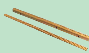
Modelo: Cremallera con herraje Código: CR1 - Medidas: 1000 x 25 x 20
