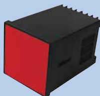
Modelo: 96 x 96 para bornes Código: 9696B - Medidas: 96 x 96 x 145
