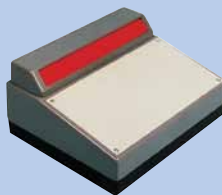
Modelo: PC60 con visor - Código: PC60CV/04/6 - Medidas: 232 x 192 x 114
