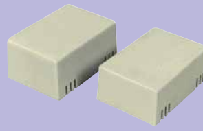
Modelo: P06N/1 Vent. Código: P06N/1/03/6 Medidas: 64 x 44 x 30 Modelo: P07N Vent. Código: P07NV/1/00/6 Medidas: 64 x 44 x 25
