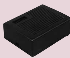
Modelo: P12 - Código: P12/00/6 - Medidas: 102 x 82 x 37
