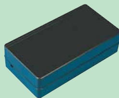
Modelo: FW3 - Código: FW3/00/6 Medidas: 136 x 73 x 37
